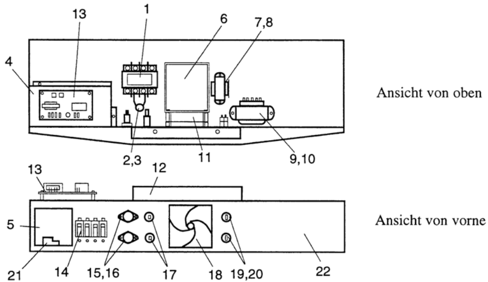
DZ33II Elektrokonsole
