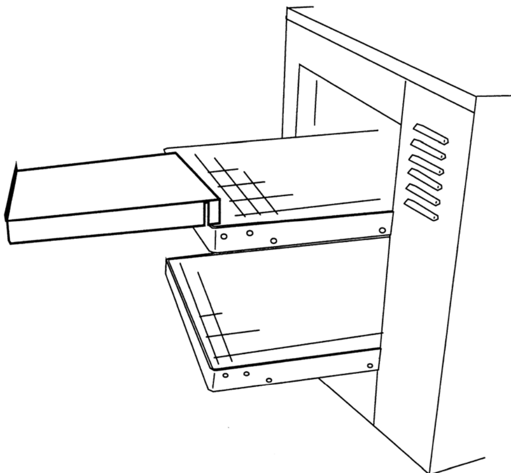
Abbildung 2-14 Installation der Ausgangsrampe
