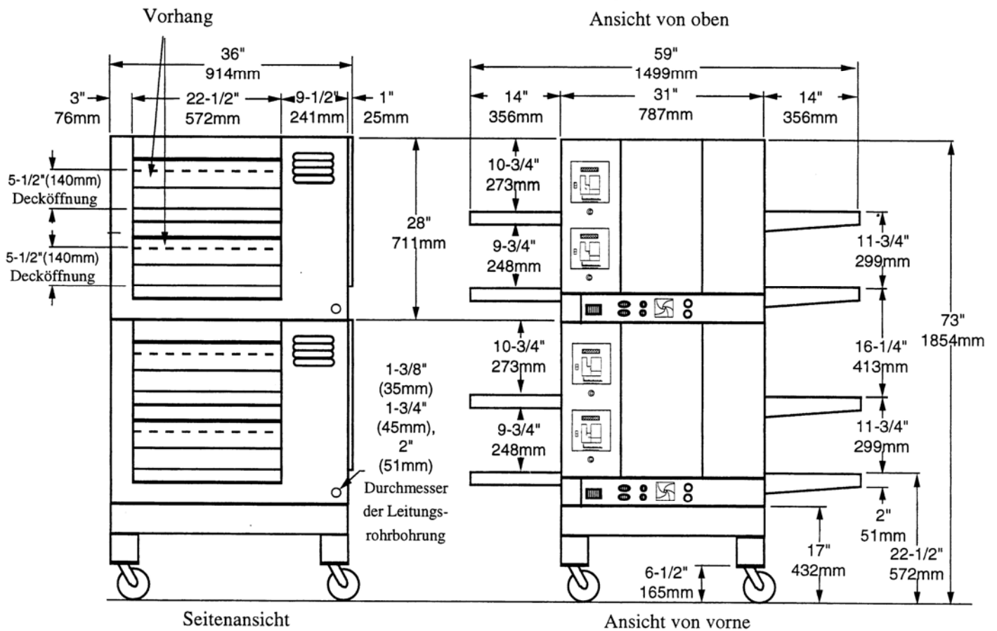
Ofen DZ33II, Doppelausführung auf Gestell mit zwei MenuSelect-Regelungen/Ofen
