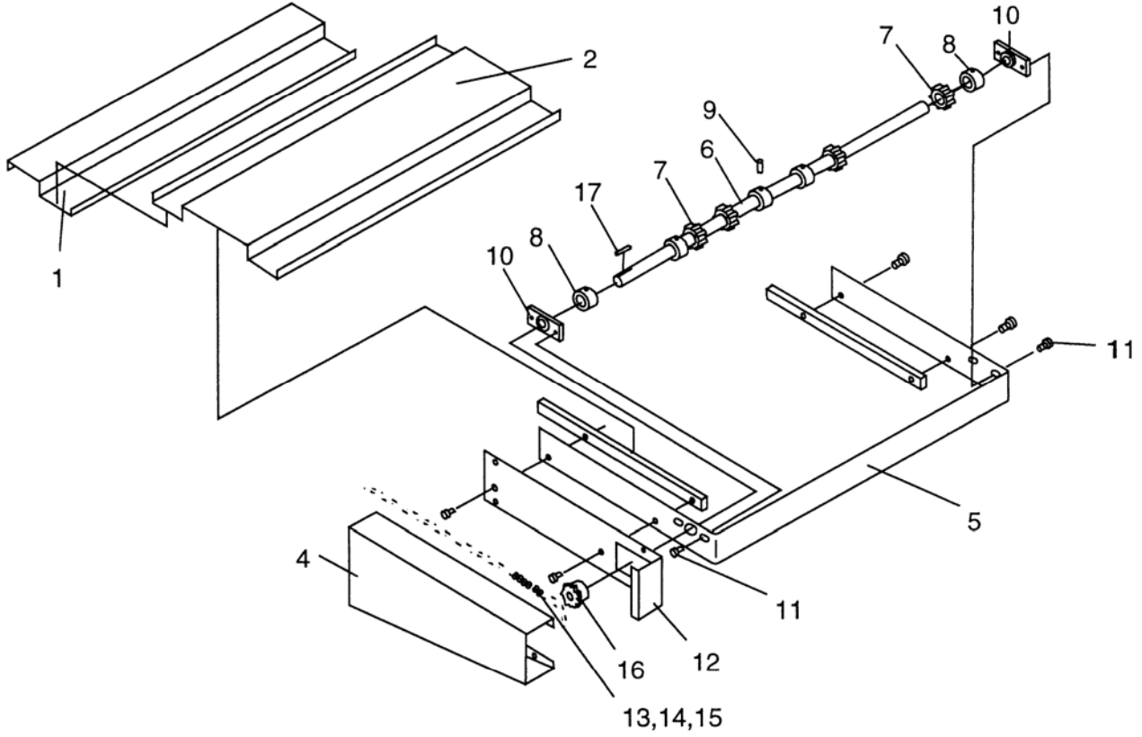
Abbildung 6-2 Antriebswelle und Umlenkrollenwelle
