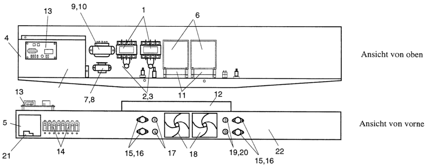
DZ5II Elektrokonsole
