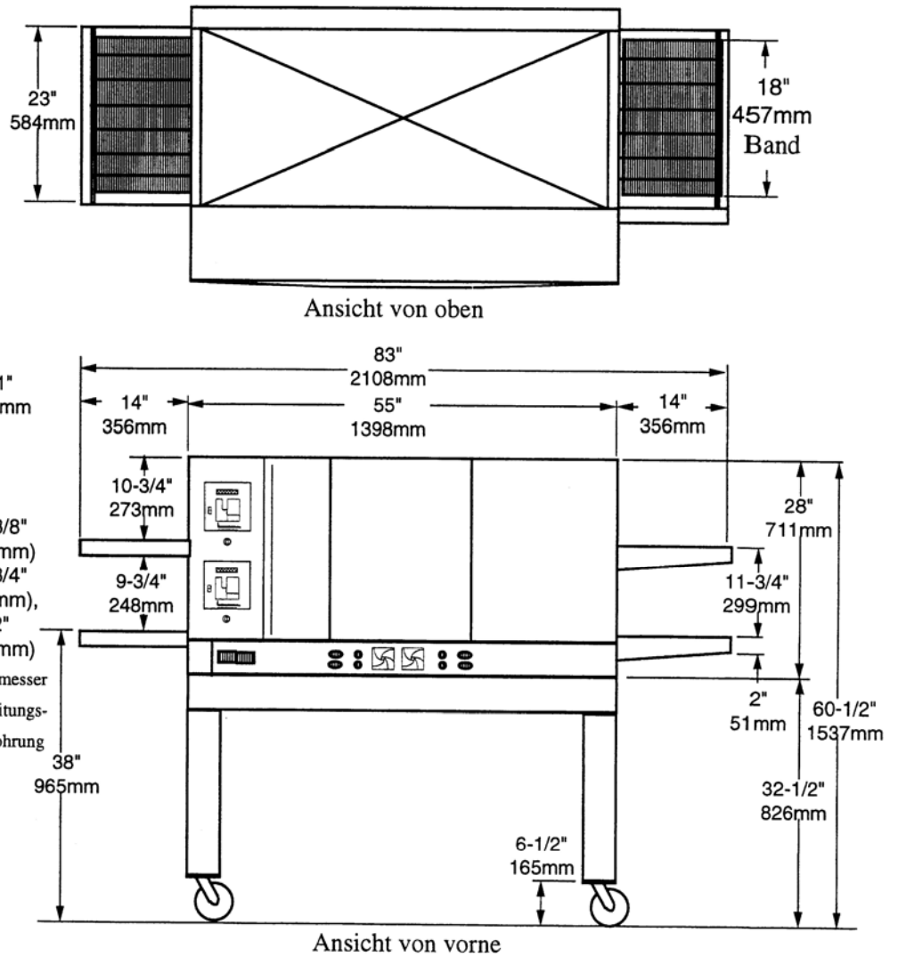
Ofen DZ55II, Einzelausführung auf Gestell mit zwei MenuSelect-Regelungen
