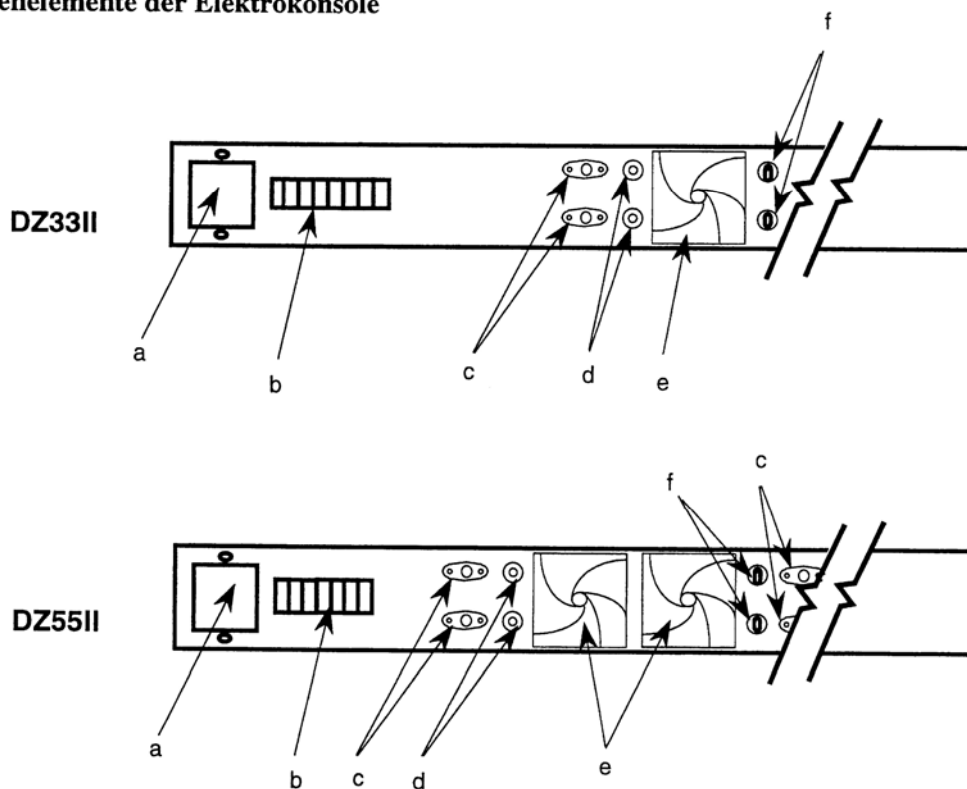
Abbildung 3-2 Elektrokonzole
