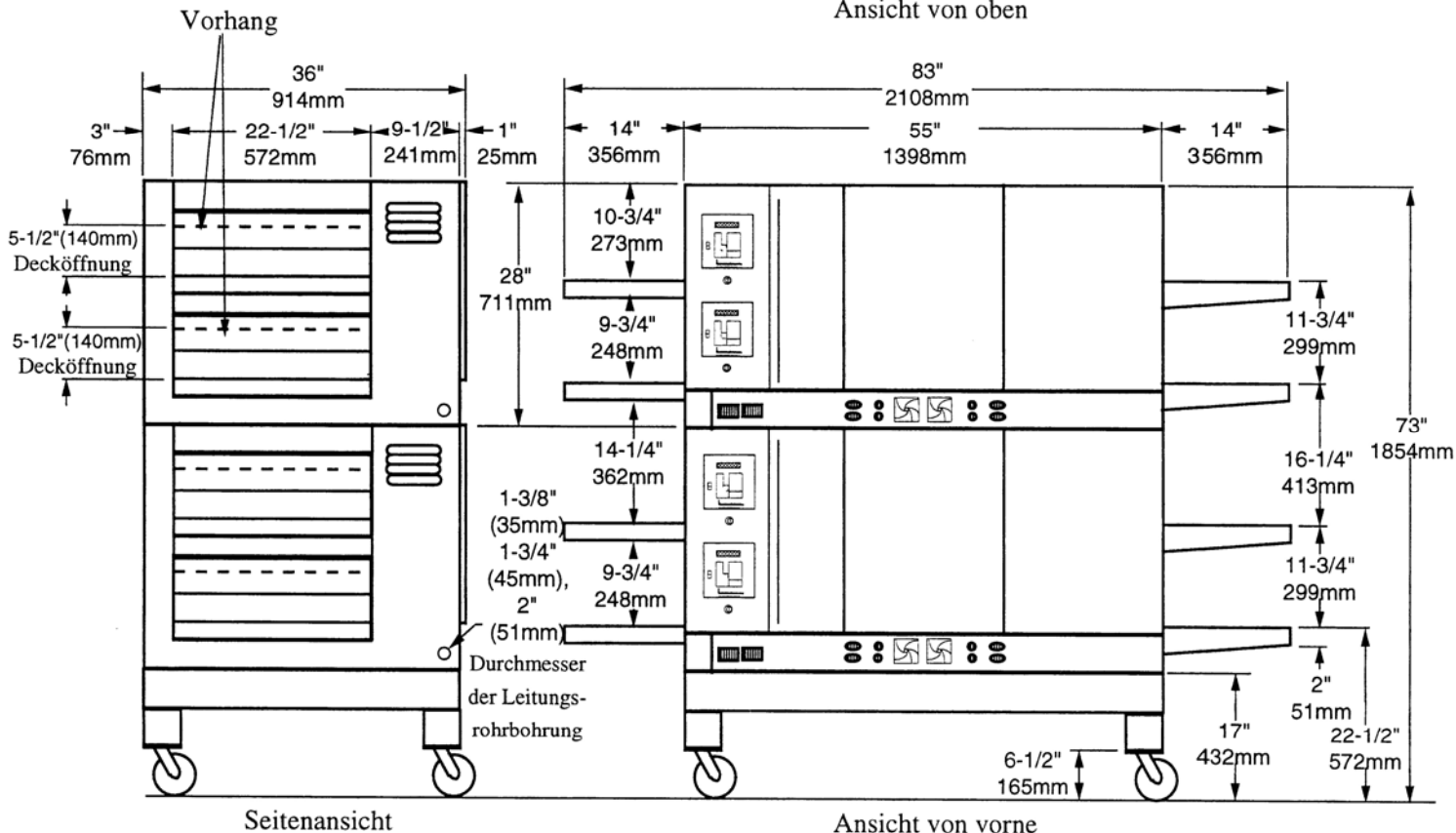
Ofen DZ55II, Doppelausführung auf Gestell mit zwei MenuSelect-Regelungen/Ofen
