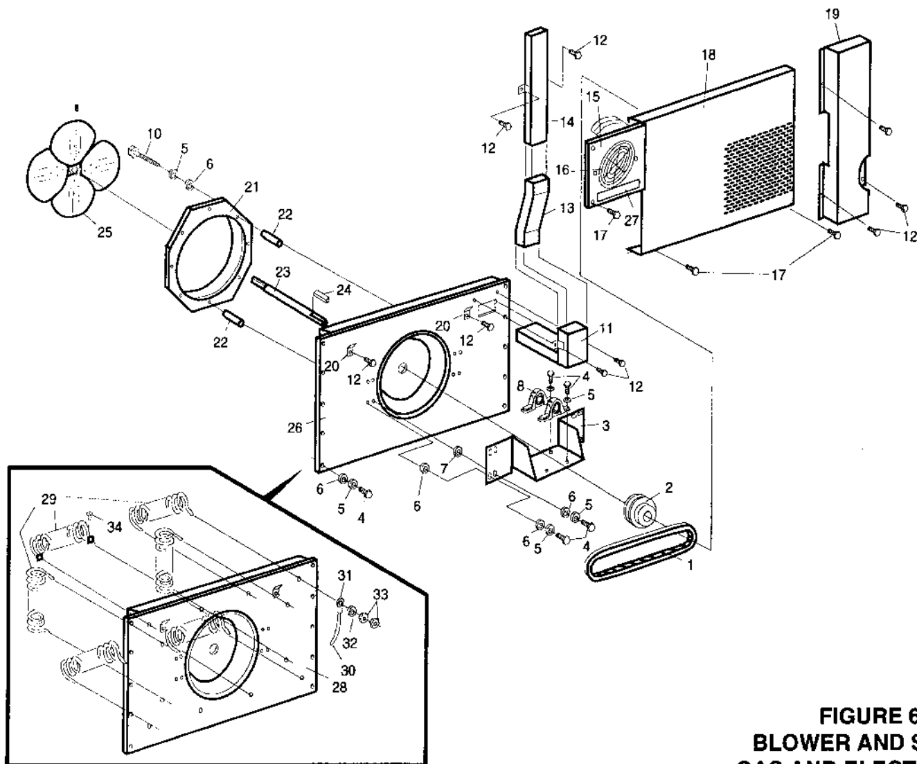
FIGURE 6-4 SOUFFLERIE ET TÔLE DE PROTECTION DES FOURS À GAZ ET ÉLECTRIQUES
