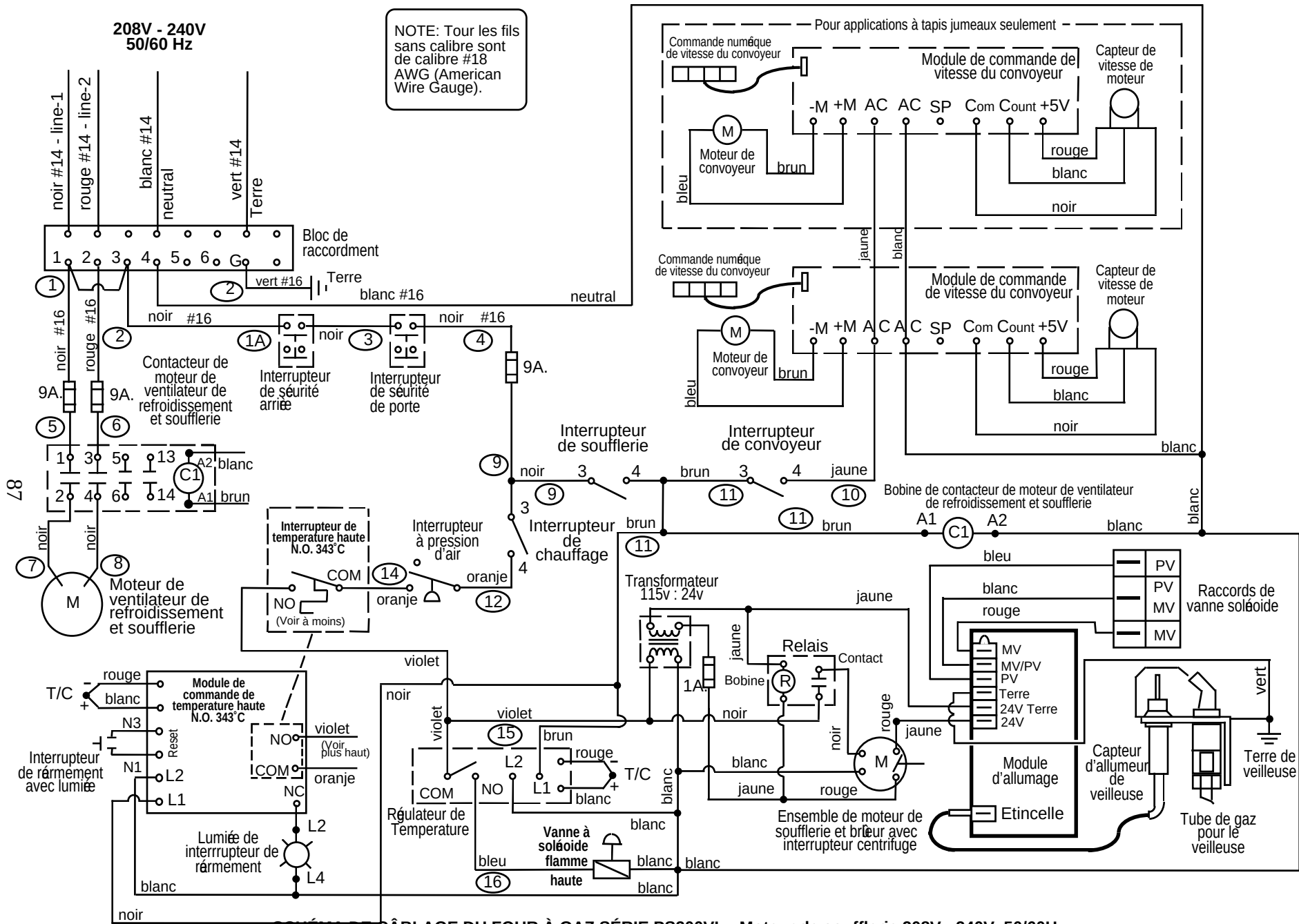
SCHEMA DE CÂBLAGE DU FOUR À GAZ SÉRIE PS200VL : Moteur de soufflerie 208V - 240V, 50/60Hz, 4,1A, tripolaire, 4 fils, (2 conducteurs, 1 neutral, 1 terre), monophasé, Circuit de commande 120V
