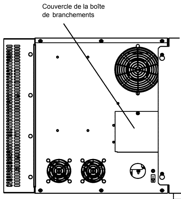
Figure 2-12. Boîte de branchements
