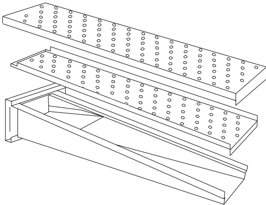
Figure 4-14. Doigts pneumatiques supérieurs standards
