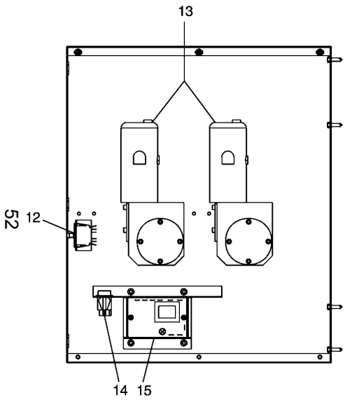
Boîte de contrôle intérieure du mur frontal
