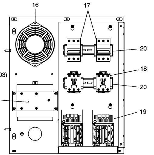
Boîte de contrôle intérieure du mur postérieur
