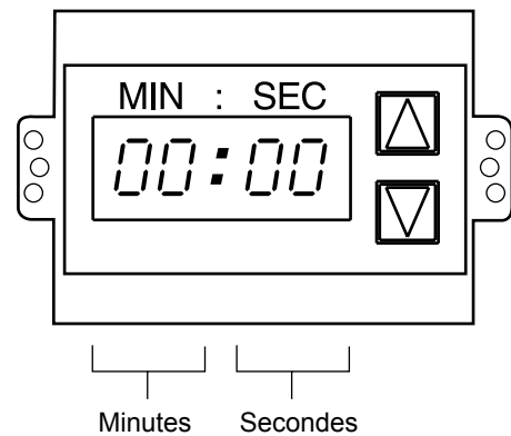
Figure 3-3. Contrôle numérique de vitesse du transporteur
