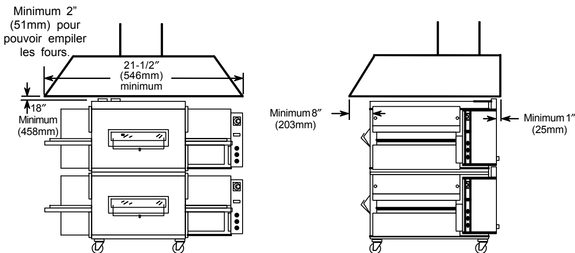
Figure 2-10. Hotte d'extraction
