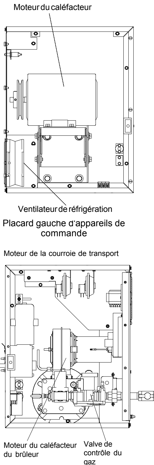
Placard droit d'appareils de commande
