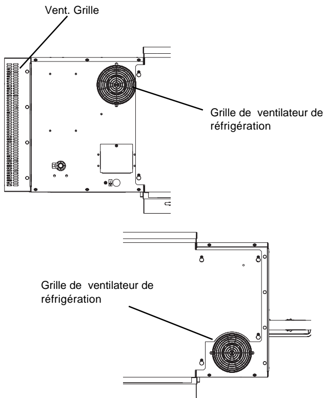
Figure 4-1. Ventilateurs de réfrigération du four
