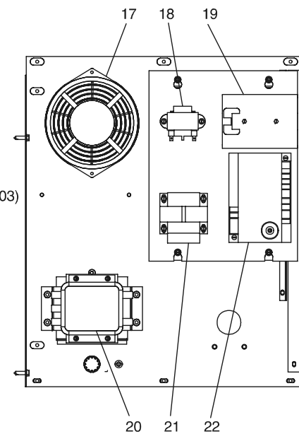
Boîte de contrôle intérieure du mur postérieur
