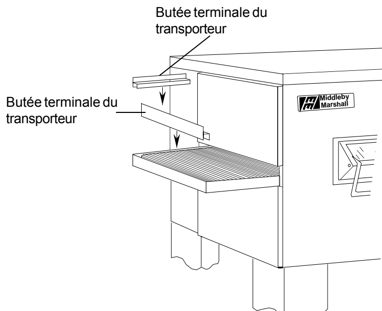
Figure 2-14. Installation des butées postérieures et terminales
