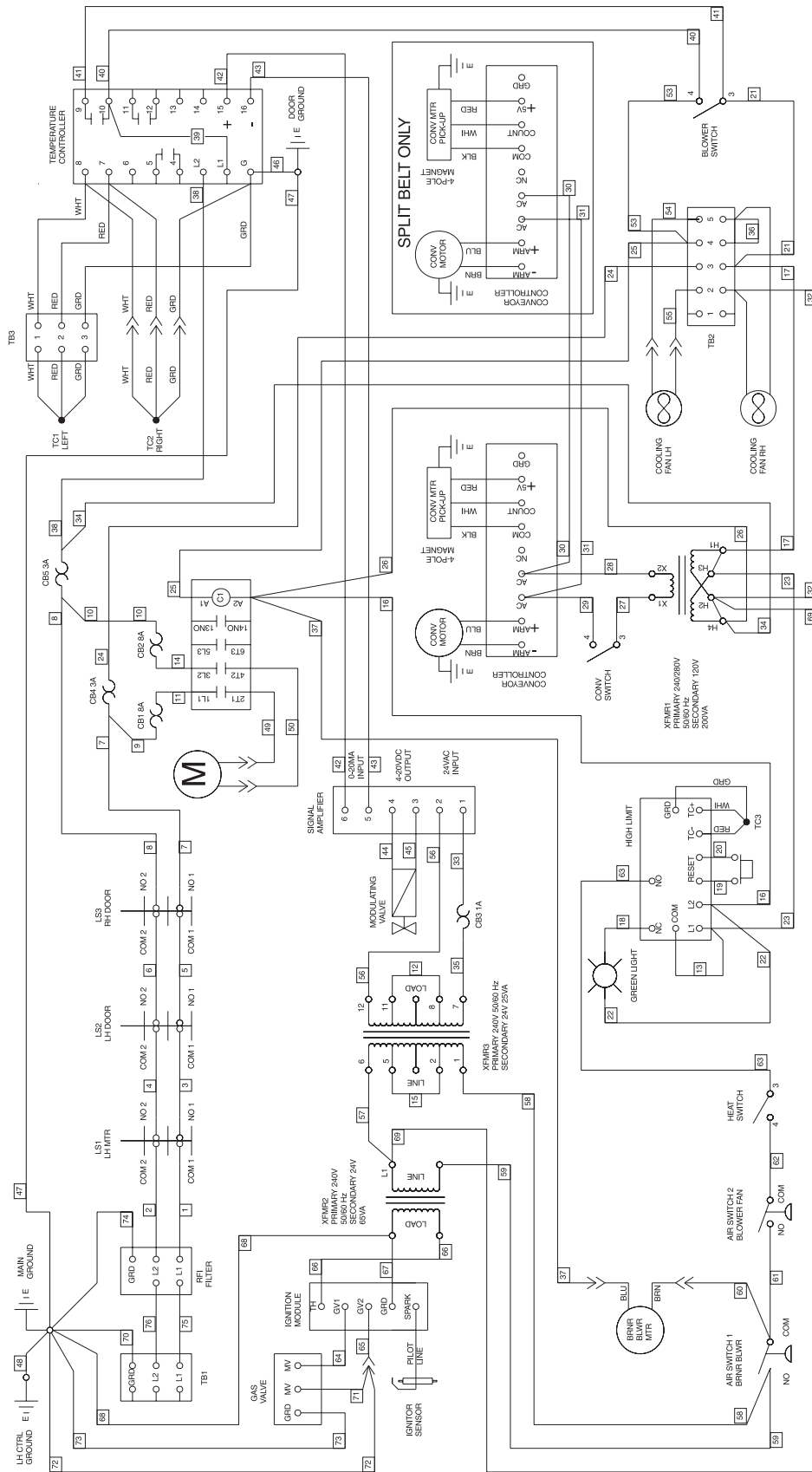
Diagramme du câblage, G208-240 50/60, 1PH 3W PS540
