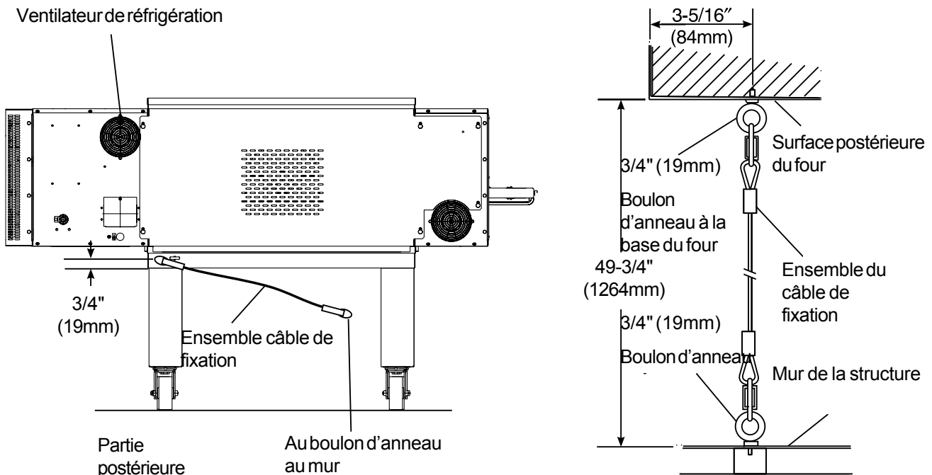
Figure 2-8. Installation de l'ensemble de câble de fixation
