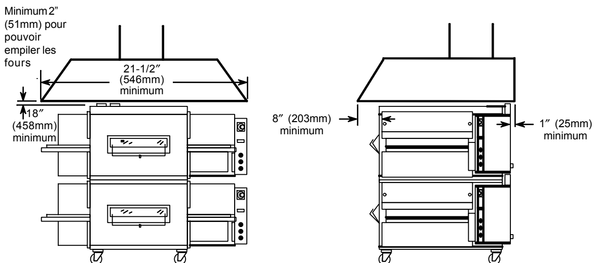
Figure 2-10. Hotte d'extraction
