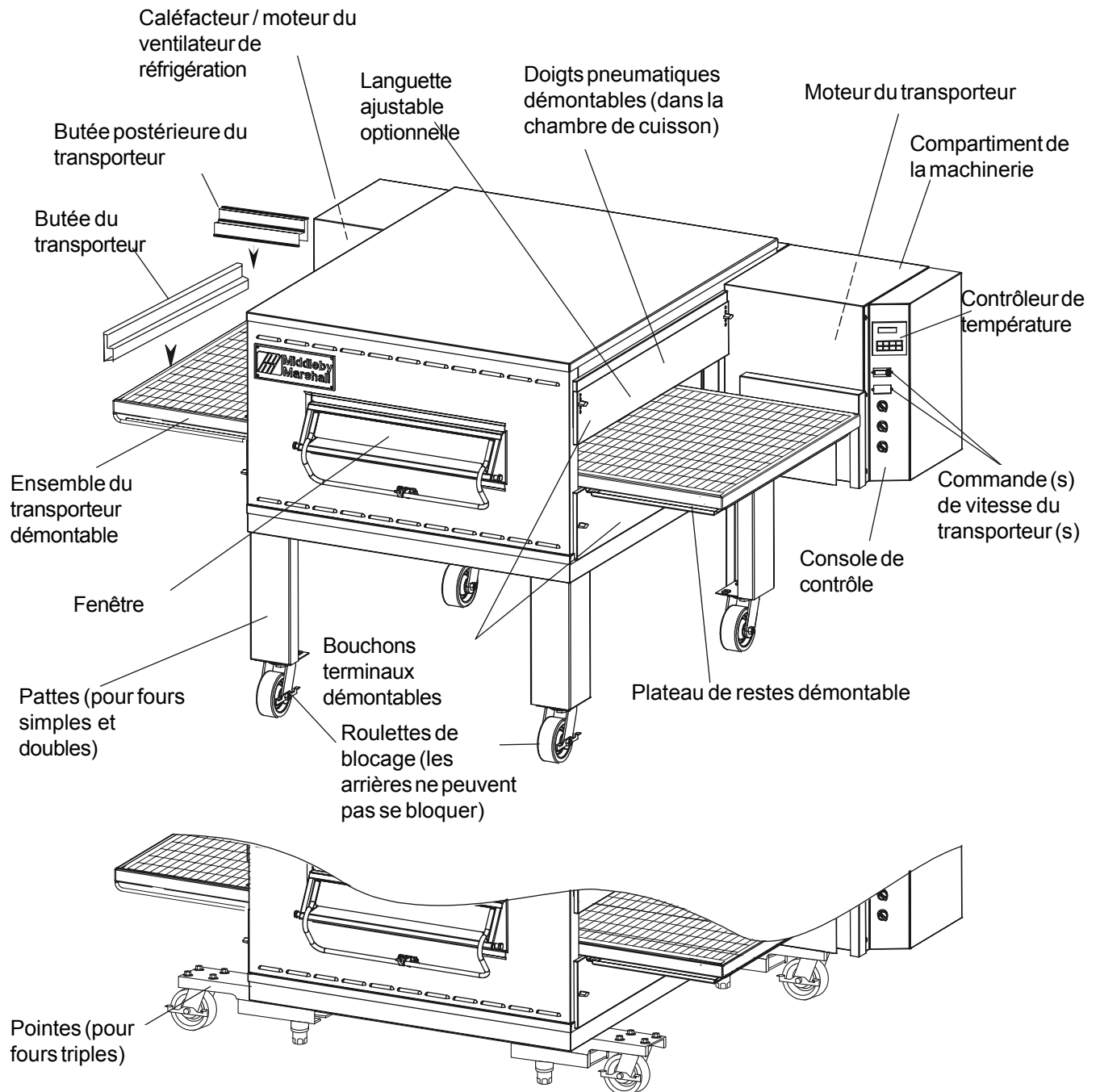
Figura 1-6. Situation des composants du four de la série PS540
