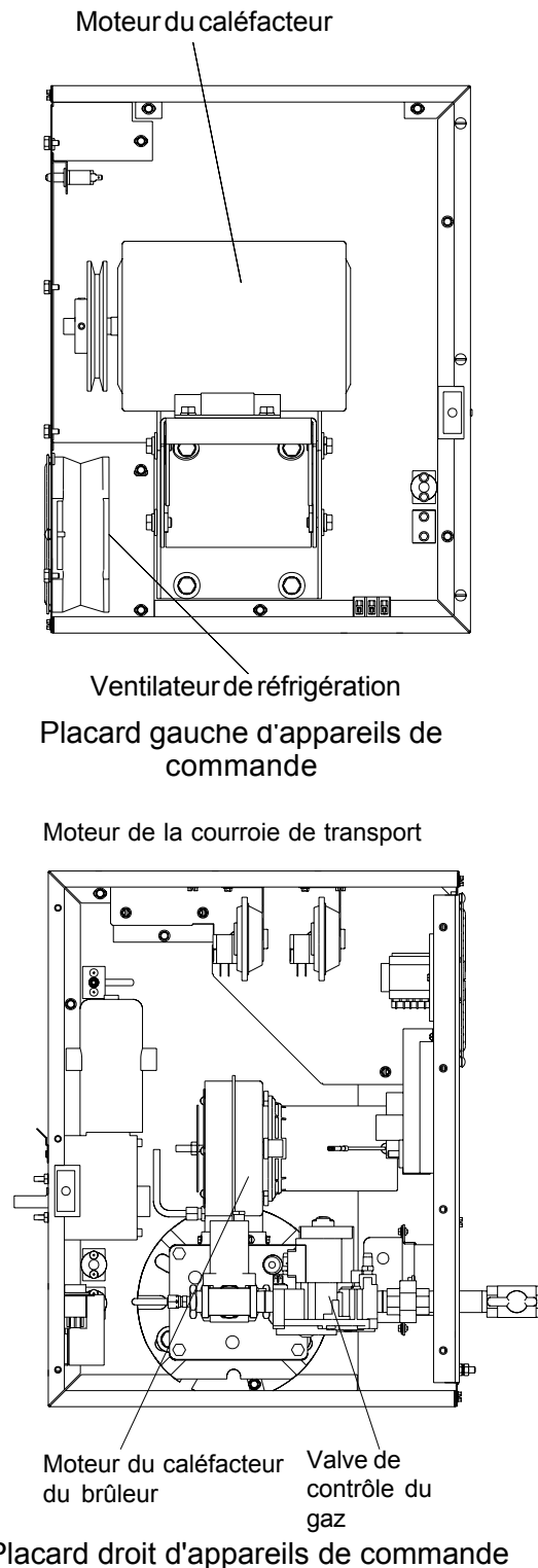
Figure 1-7. Composants du compartiment de la machinerie
