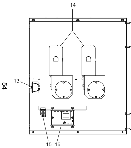
Boîte de contrôle intérieure du mur frontal
