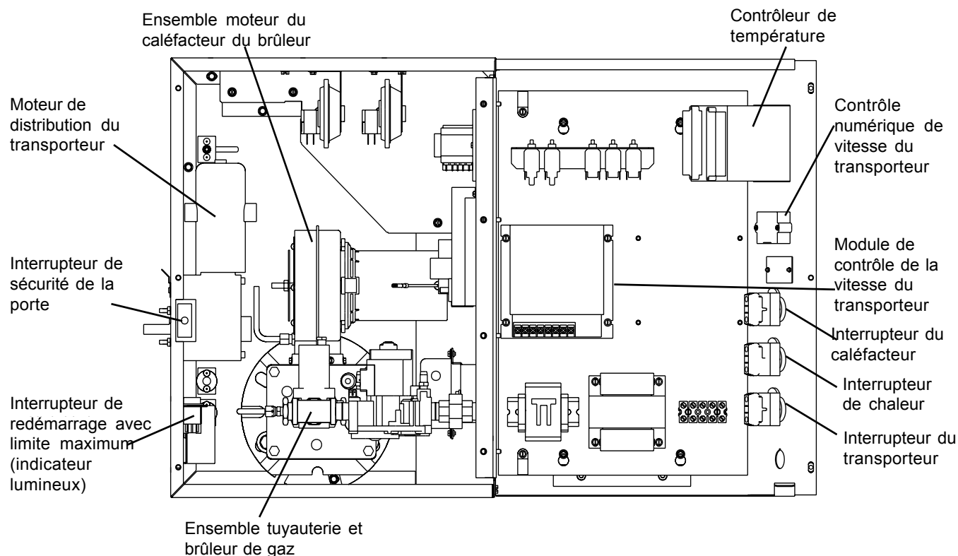
Figure 3-2. Vue intérieure du compartiment de machinerie et de la console de commandes
