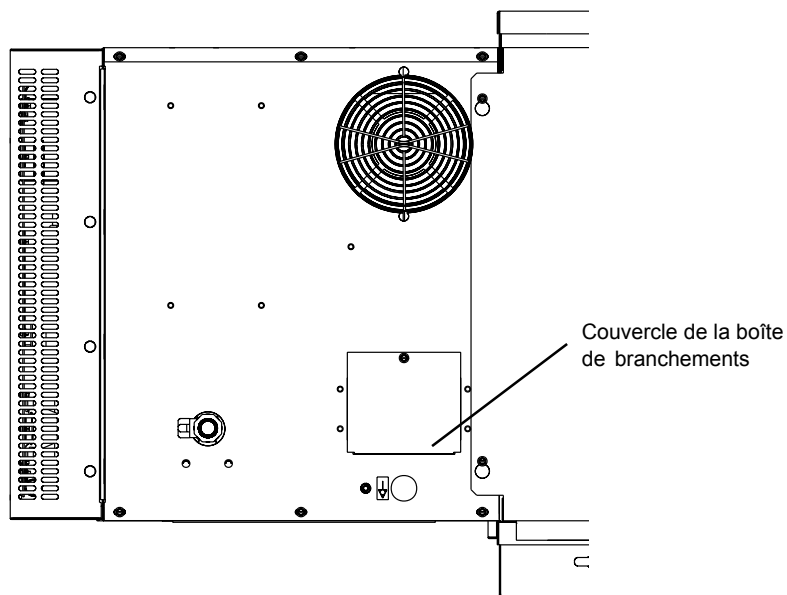
Figure 2-12. Boîte de branchements
