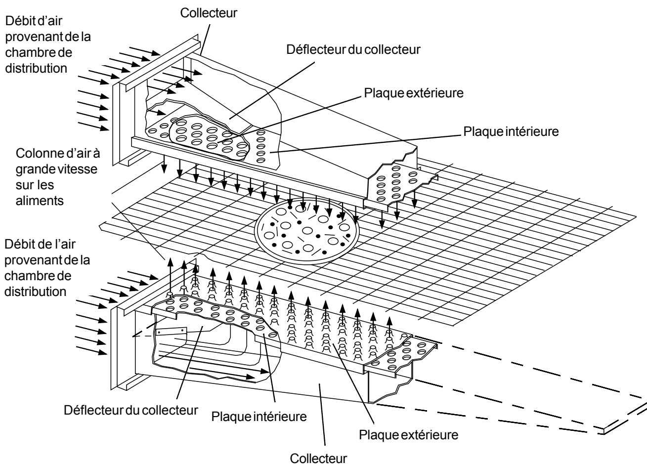
Figure 1-5. Doigts pneumatiques, qui montrent les colonnes de grande vitesse de l'air qui se forment en passant par la plaque extérieur et la plaque intérieure pour chauffer l'aliment.
